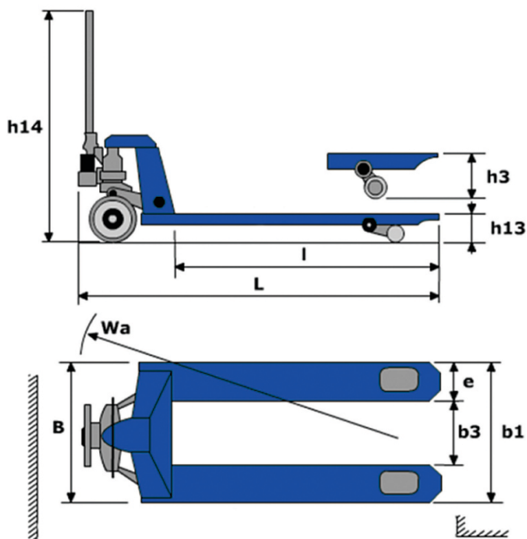
Рисунок 1 - Габаритные размеры весов
